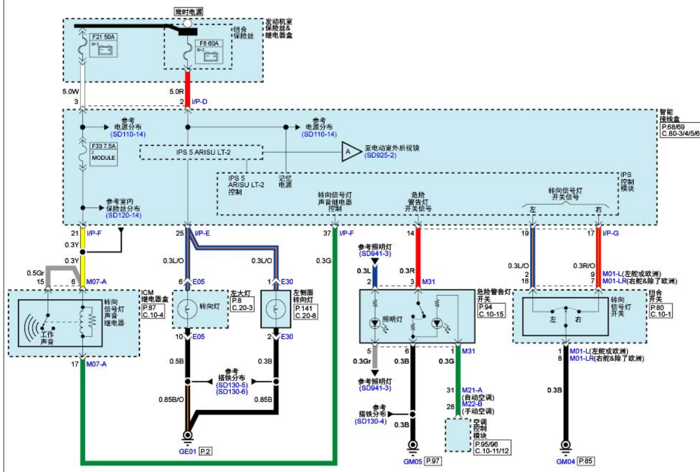
转向灯&amp;危险警告灯(1)
